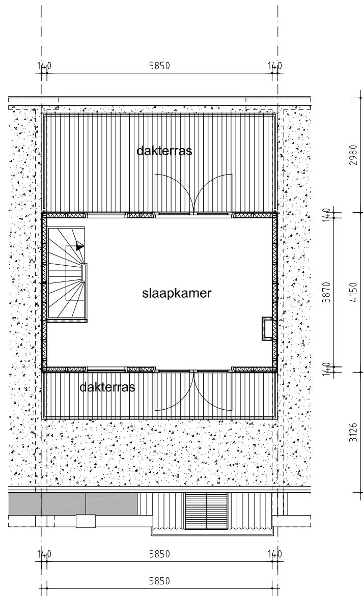
dakverdieping
