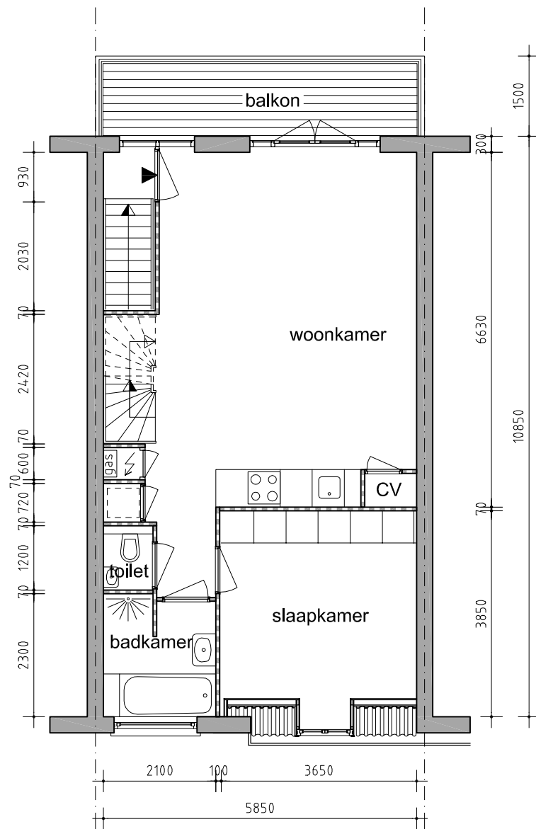
2e verdieping
